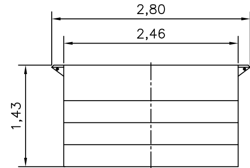
VISTA - 'B'
