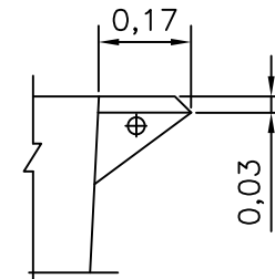
DETALHE-C ESC.1:15
