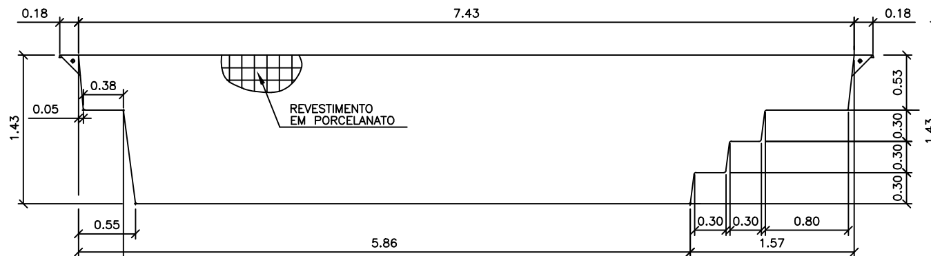
SEÇÃO A-A
