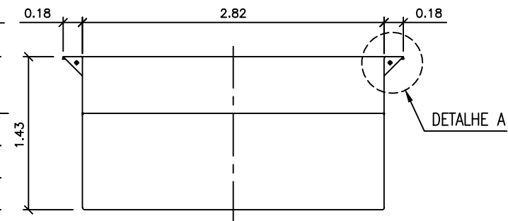
SEÇÃO B-B
