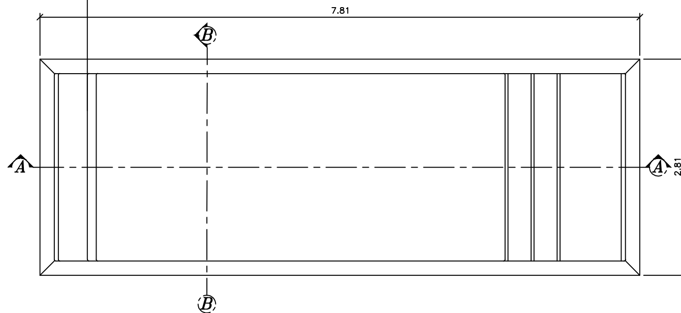
PLANTA BAIXA
