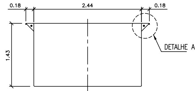
SEÇÃO B-B
