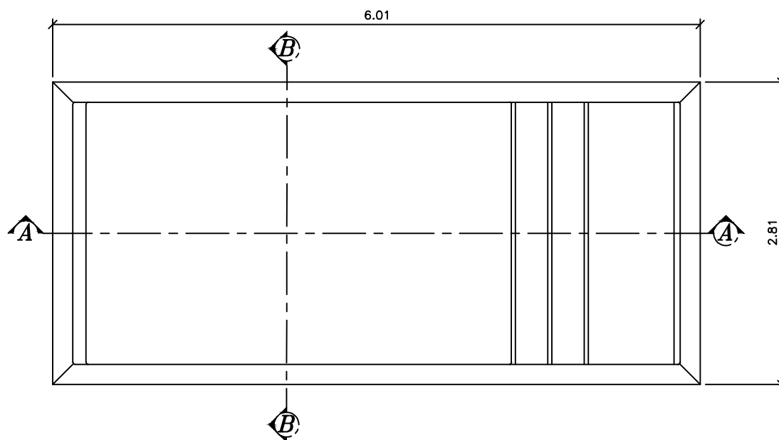
PLANTA BAIXA
