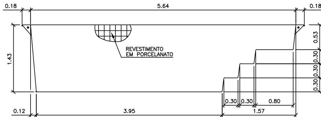
SEÇÃO A-A
