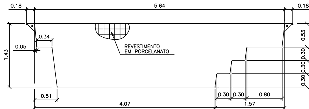
SEÇÃO A-A
