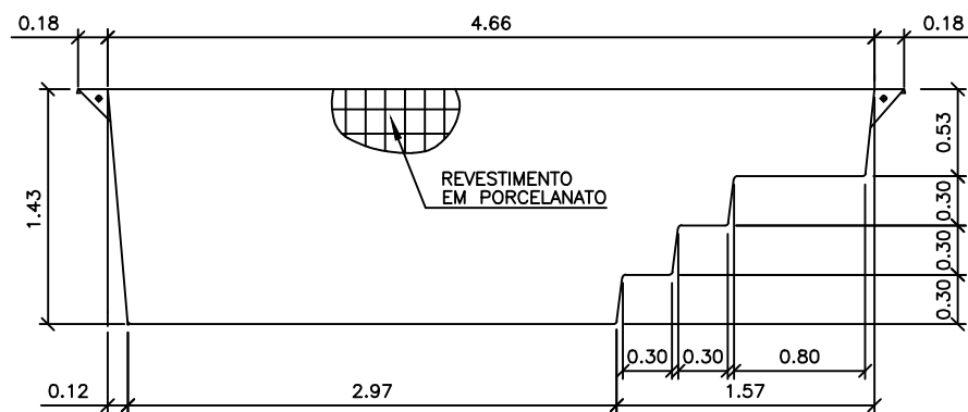
SEÇÃO A-A
