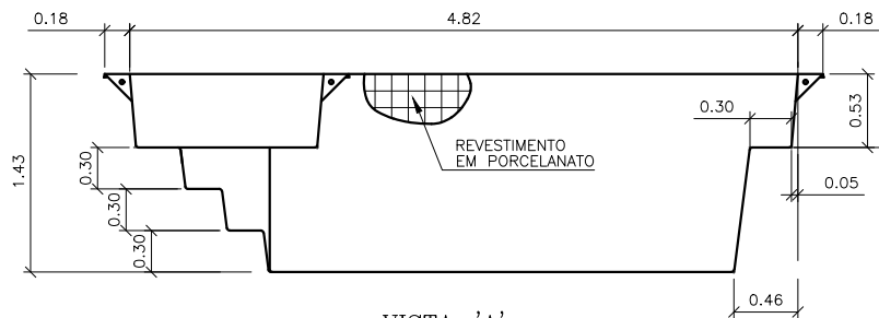
VISTA - 'A'
