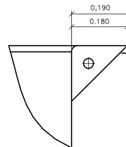
DETALHE - C ALÇA DE IÇAMENTO ESC. 1=10
