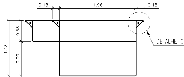
VISTA - 'B'
