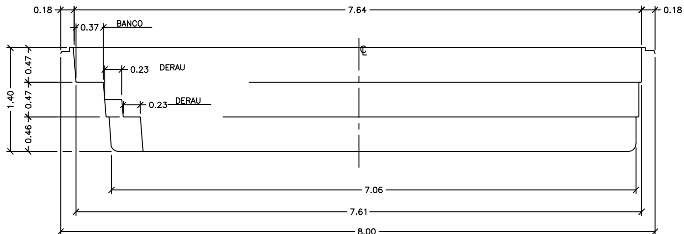
Seção - AA
