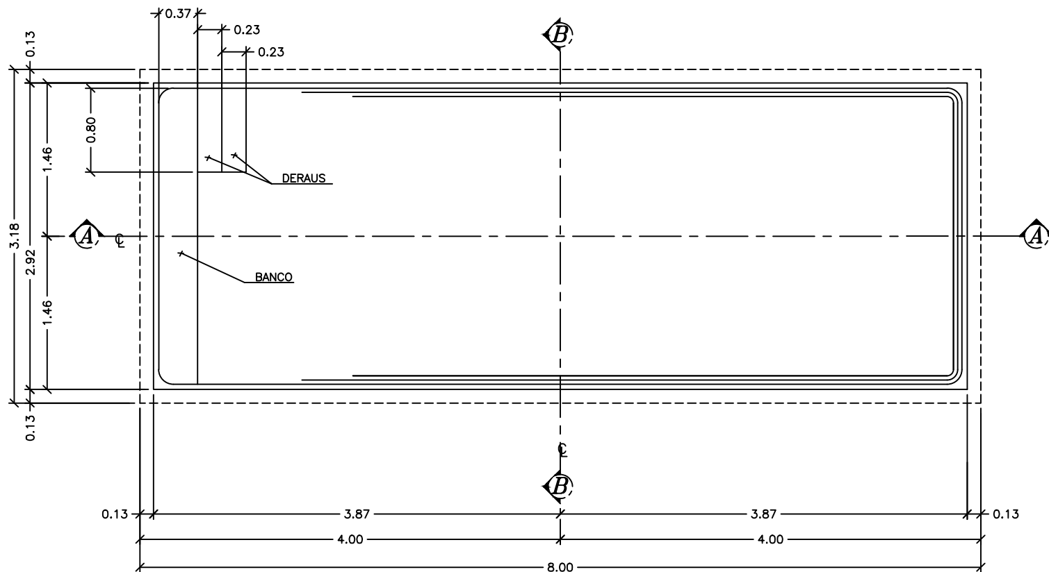
Planta Baixa
