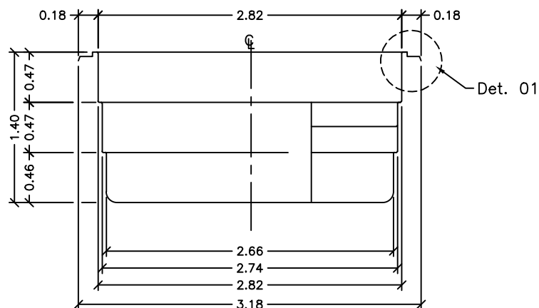
Seção - BB
