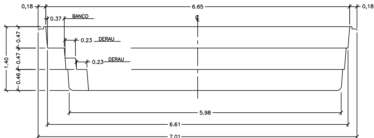
Seção – AA
