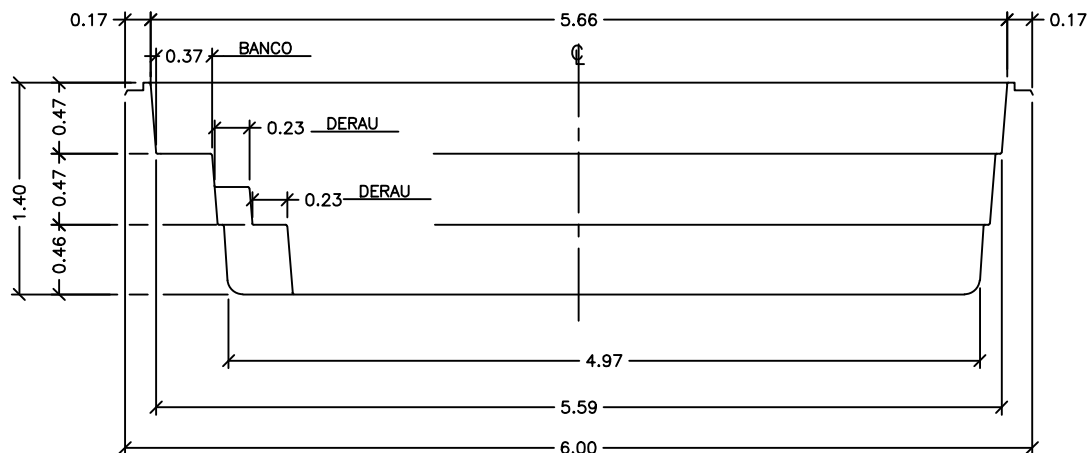
Seção - AA
