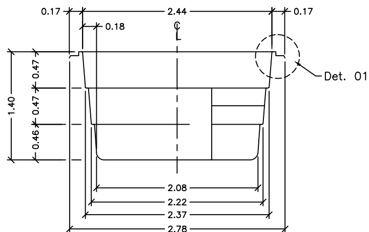
Seção - BB
