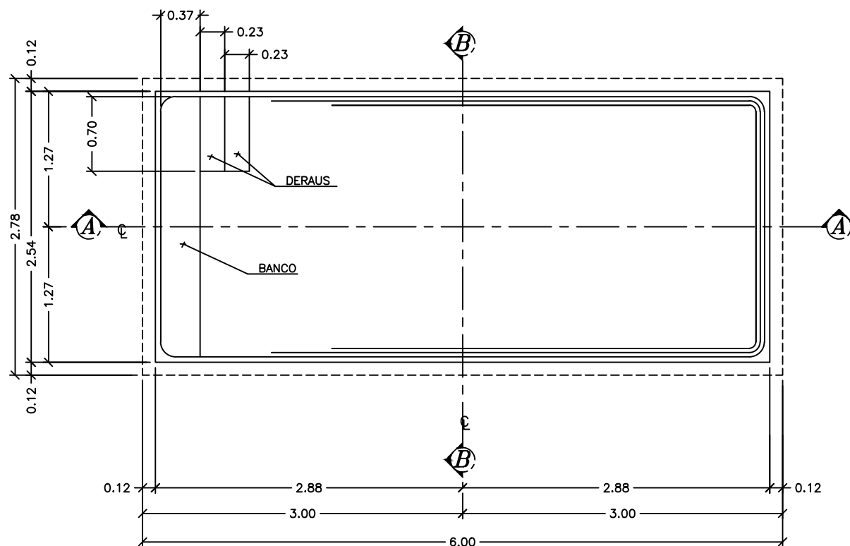
Planta Baixa
