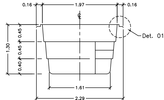
Seção - BB
